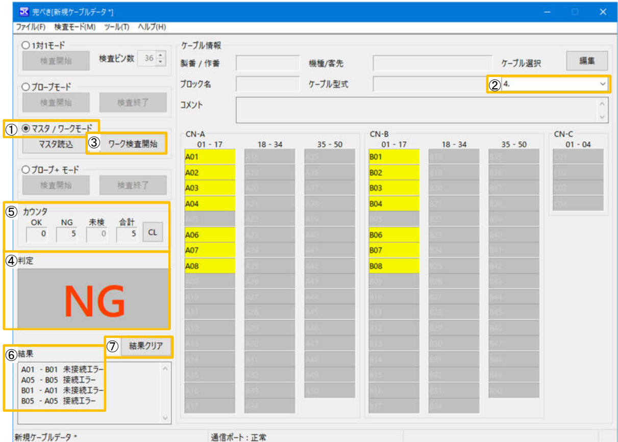
図 4-8 ワーク検査
